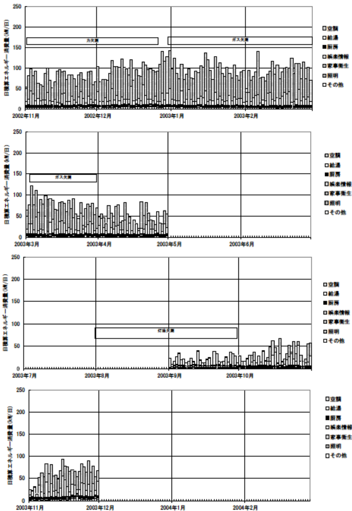
日積算エネルギー消費量 (2002年11月～2004年1月)(北海道戸建05)
