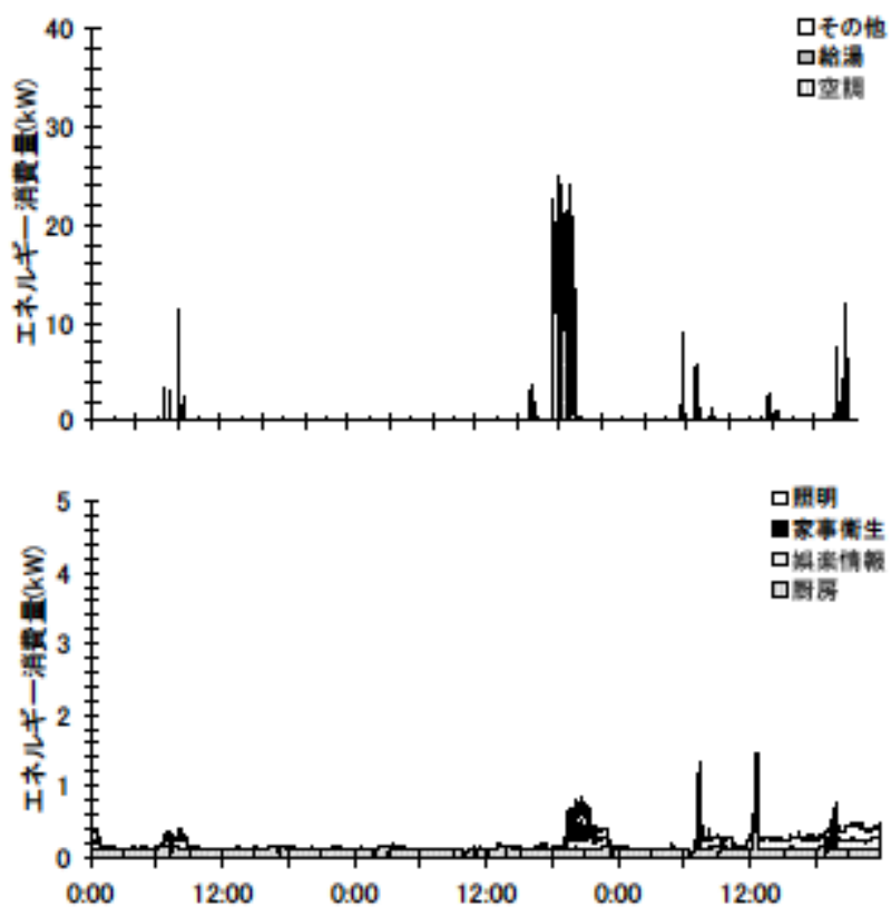
夏季の大分類用途別エネルギー消費量（2003年8月5日～7日）(北海道戸建05)
