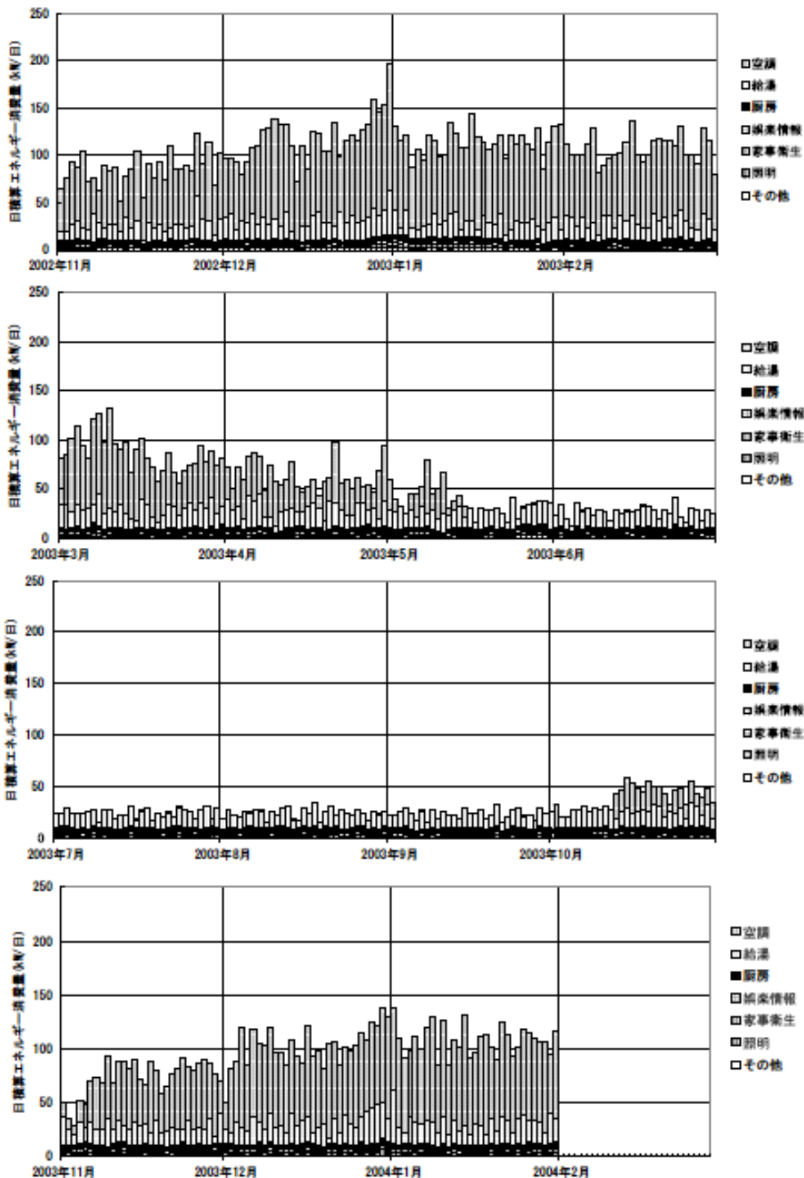
日積算エネルギー消費量 (2002年11月~2004年1月)(北海道戸建06)
