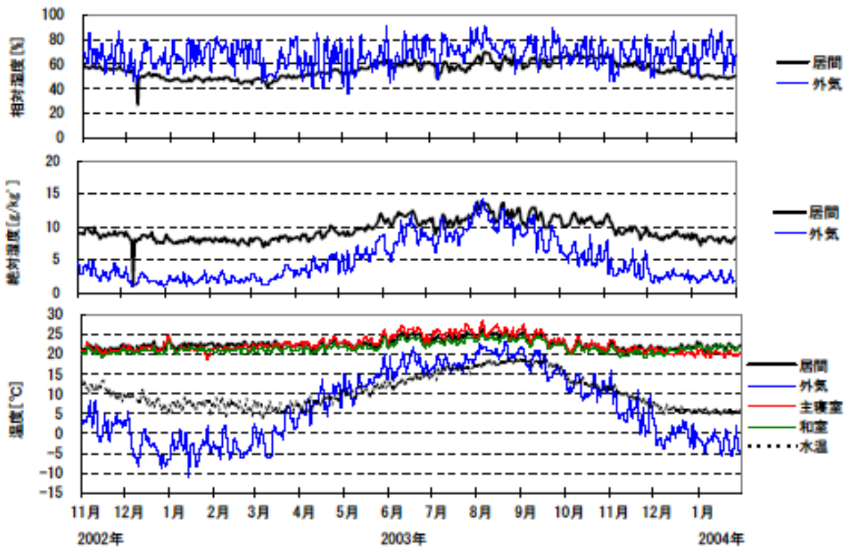
日平均温湿度 (2002年11月～2004年1月)(北海道戸建06)
