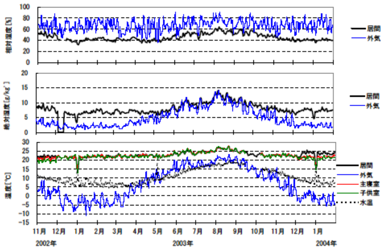
日平均温湿度 (2002年11月～2004年1月)(北海道戸建07)
