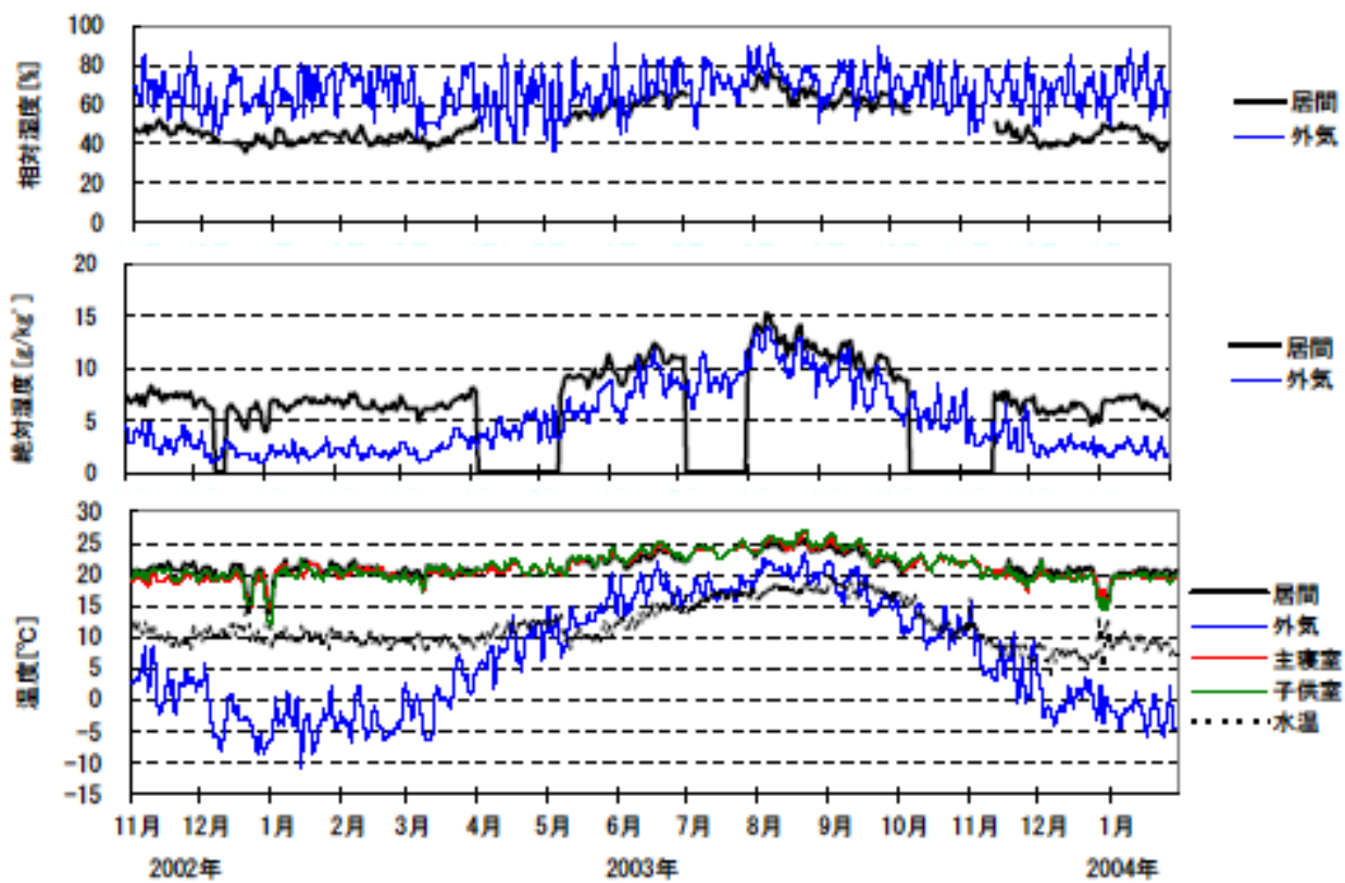
日平均温湿度 (2002年11月～2004年1月)(北海道戸建08)
