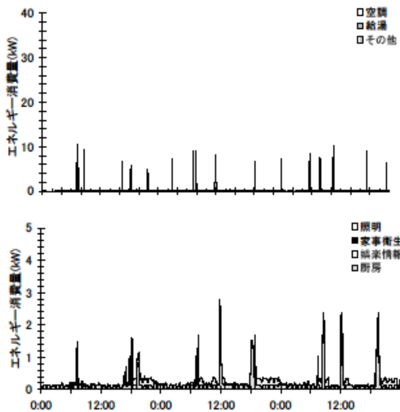
夏季の大分類用途別エネルギー消費量（2003年8月5日～7日）(北海道戸建09)
