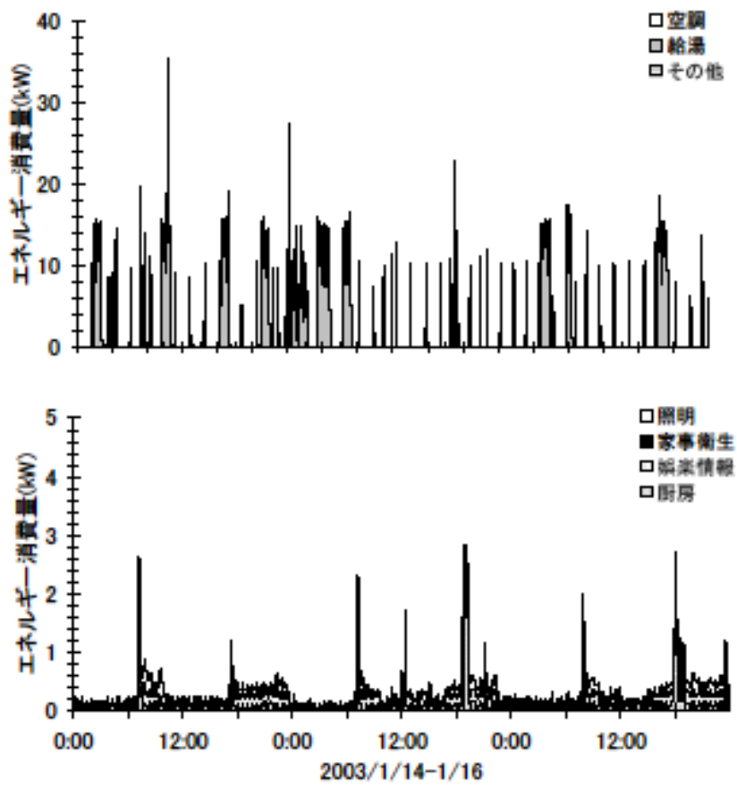
冬季の大分類用途別エネルギー消費量（2003年1月14日～16日）(北海道戸建09)
