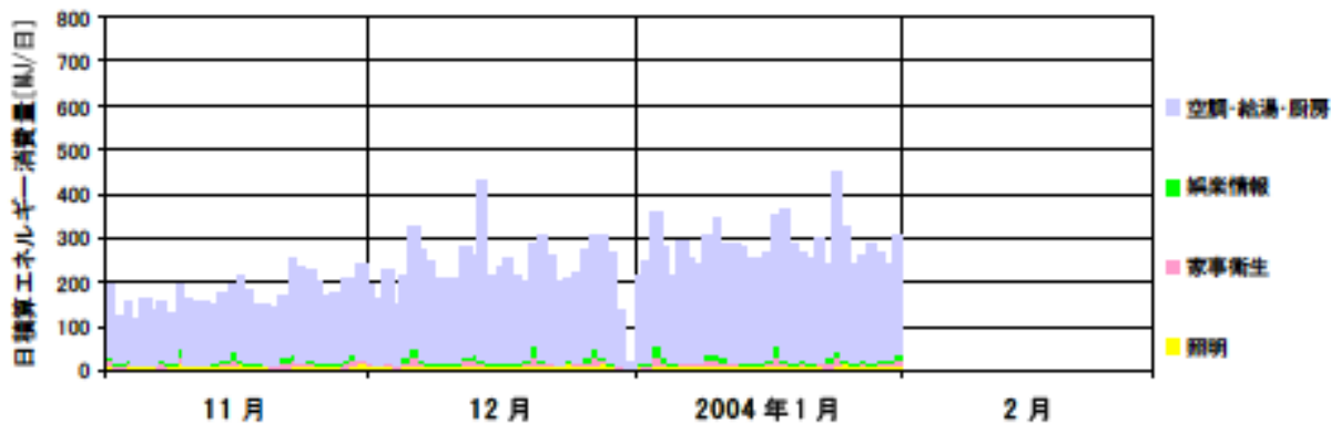
日積算エネルギー消費量 (2002年11月~2004年2月)(北陸集合 03)
