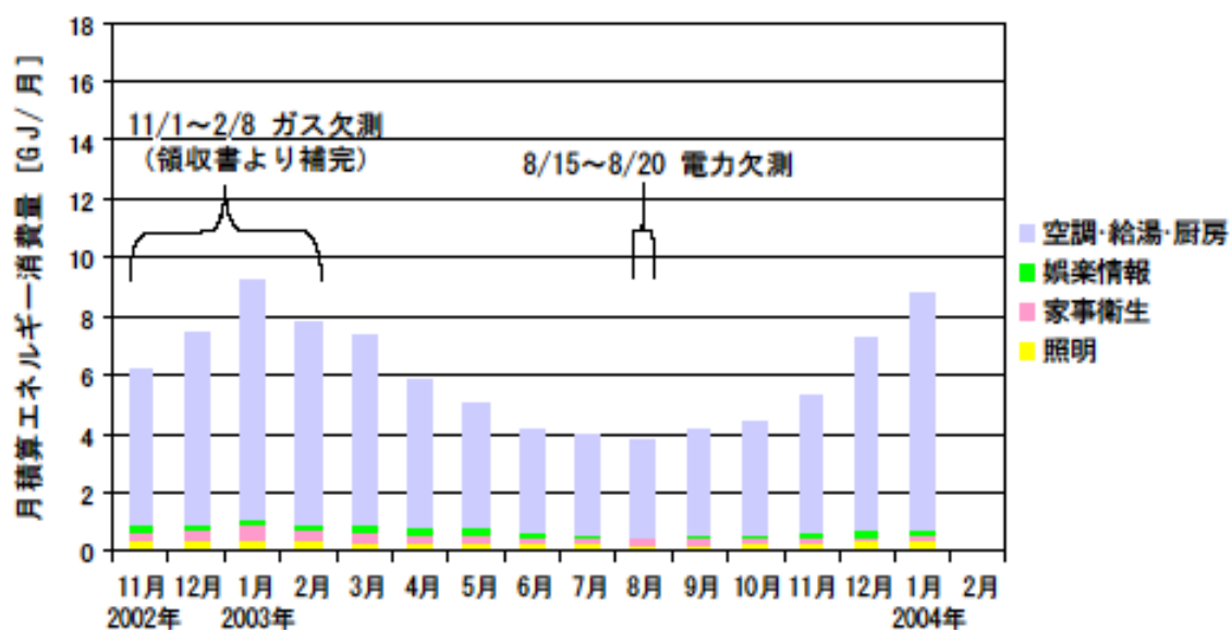
月積算エネルギー消費量 (2002年11月~2004年2月)(北陸集合 03)
