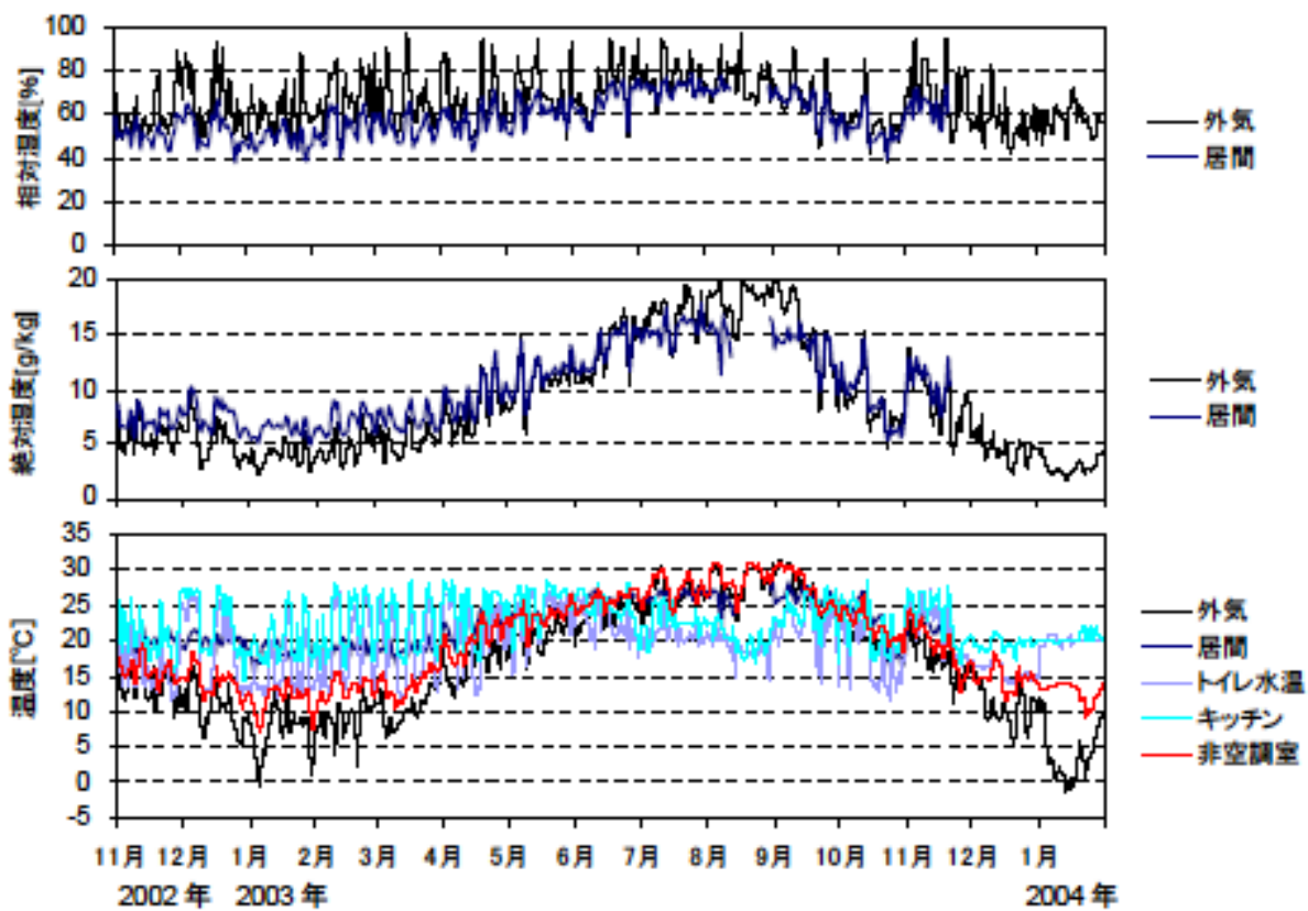
日平均温湿度 (2002年11月～2004年1月)(九州・沖縄戸建 02)
