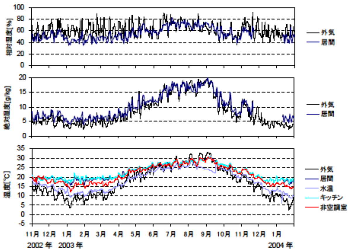
日平均温湿度 (2002年11月～2004年1月)(九州・沖縄集合 03)
