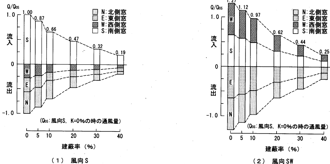
図11 建蔽率および風向の変化による各壁面窓の流入、流出風量比 (流入を+、流出を-として表示する。風向S、建蔽率0%のときの通風量で基準化する。)
