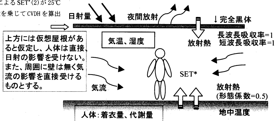
図2 人体が屋外気象条件から受ける影響
