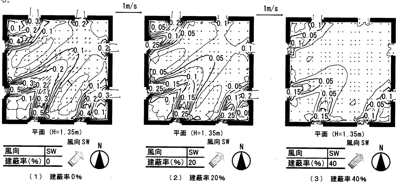
図10 室内気流分布(風向SW, 基準風速3.8m/s)
