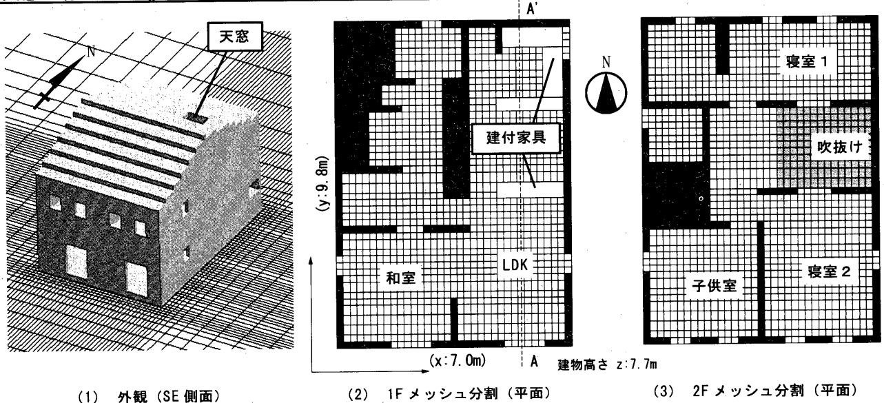
図13 実在住宅モデル
