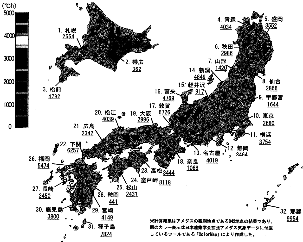
図5 全国の通風デグラワー(CVDH)マップ
