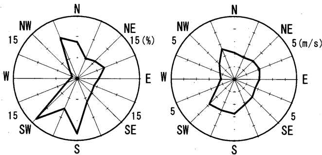
(1) 風配図 (2) 風向別平均風速
