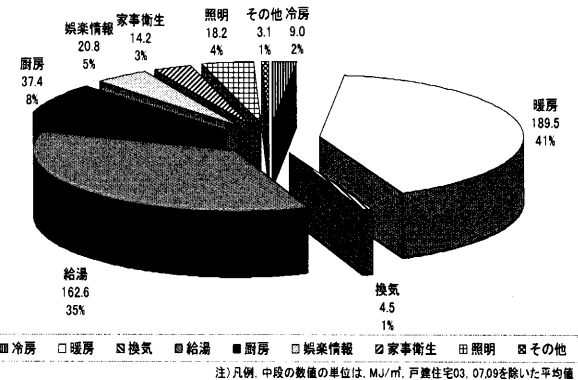
図3 戸建住宅における床面積当たりの用途別エネルギー消費量の年間積算値の平均 (2003年2月～2004年1月)
