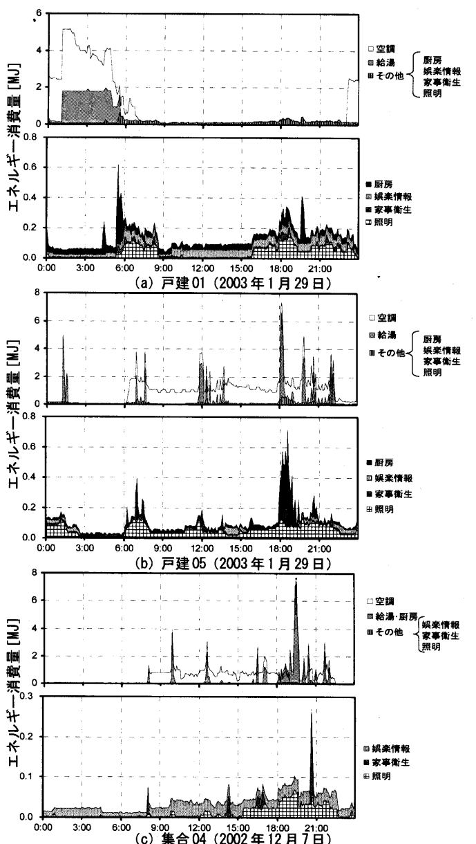
図7 最寒日における用途別エネルギー消費量の日変化
