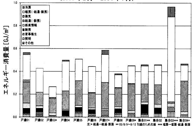
図2 床面積当たりの用途別エネルギー消費量の年間積算値 (2003年2月～2004年1月)
