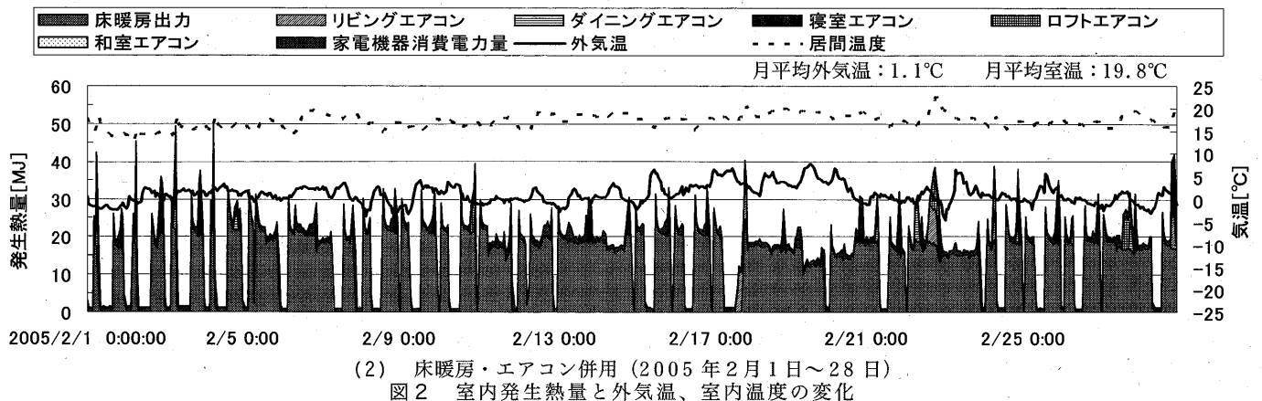
図2 室内発生熱量と外気温、室内温度の変化
