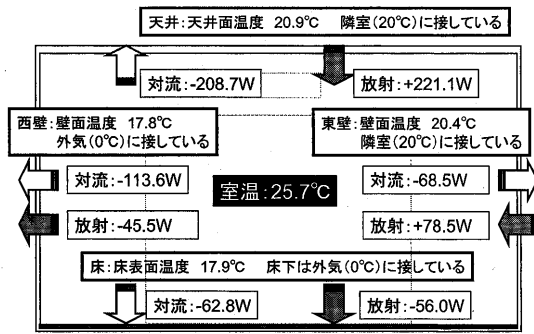
(1) 南壁から見た図 図10 温風暖房時の各壁面の放熱・受熱量および壁面温度 (case 3 エアコン吹出温度 35℃)
