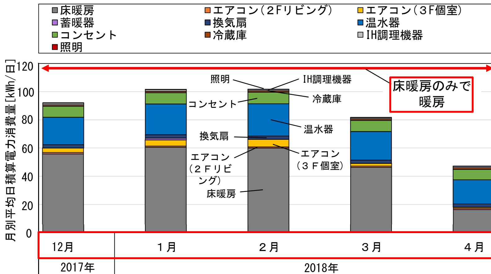
図 用途ごとの月別平均日積算電力消費量(2017年12月～2018年4月)
