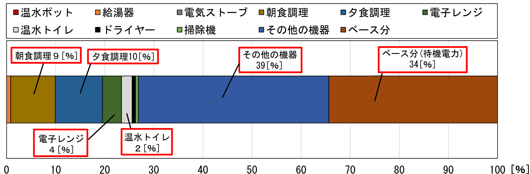
図 コンセントシステムの年積算電力消費量の割合※ 9 (2020年1月～12月)
