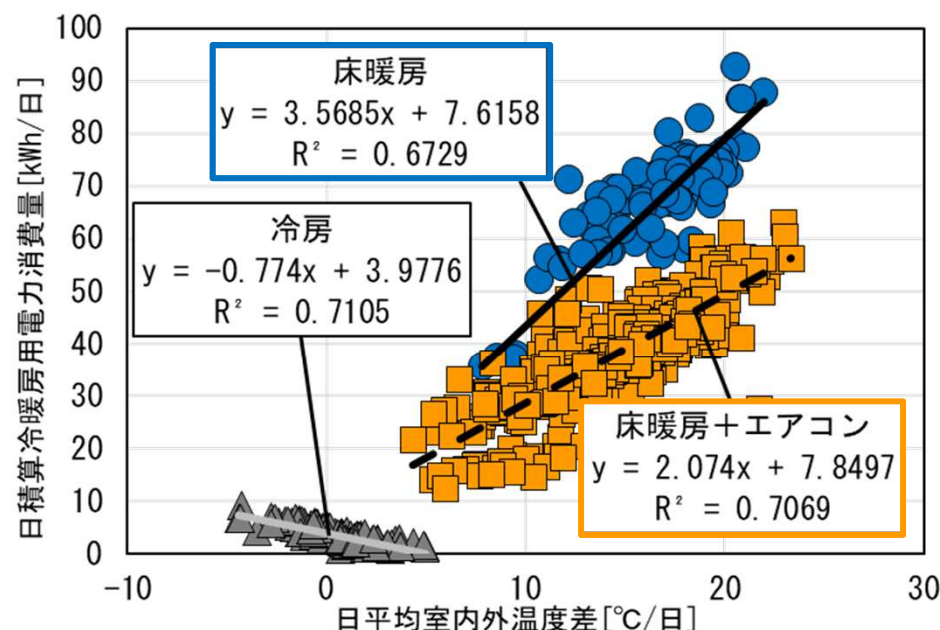
(a) 日積算冷暖房用電力消費量と 日平均室内外温度差の関係
