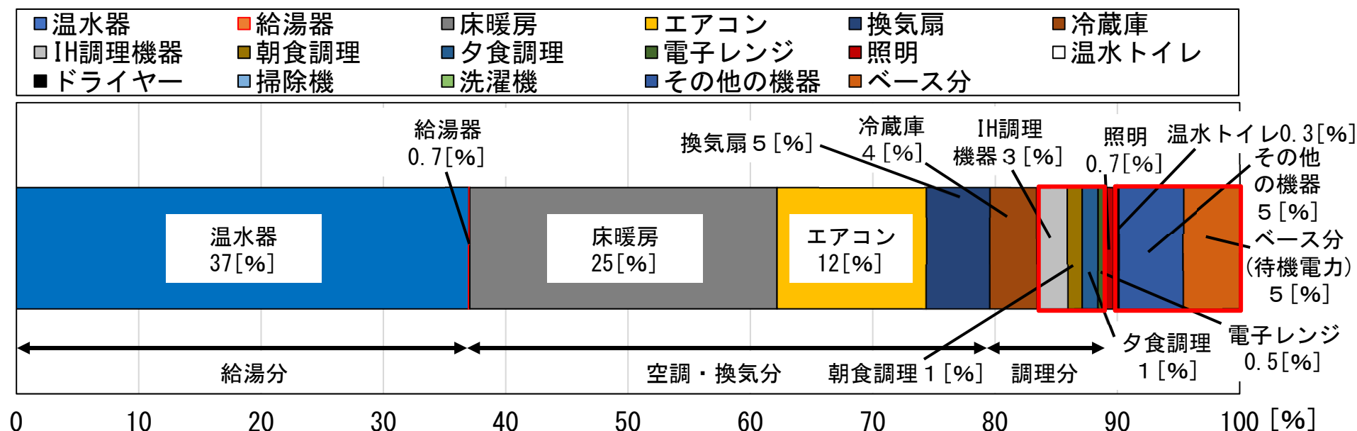
図5 用途ごとの年積算電力消費量の割合※9 (2020年1月～12月・空調方法 床暖房＋エアコン)
