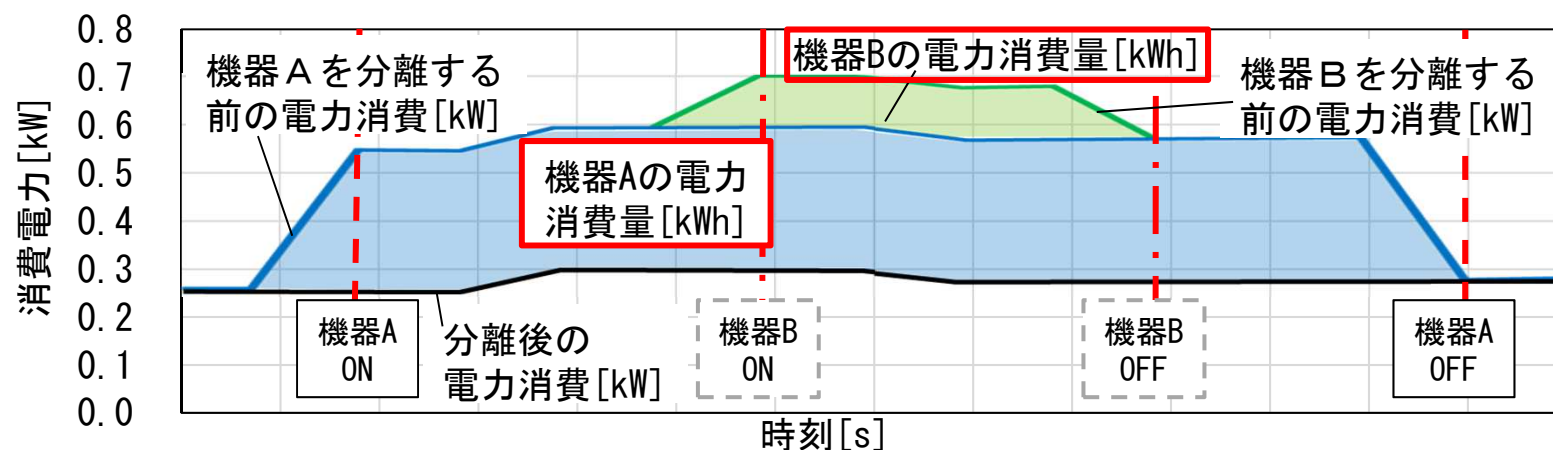
(a) 電力消費量の時間変化
