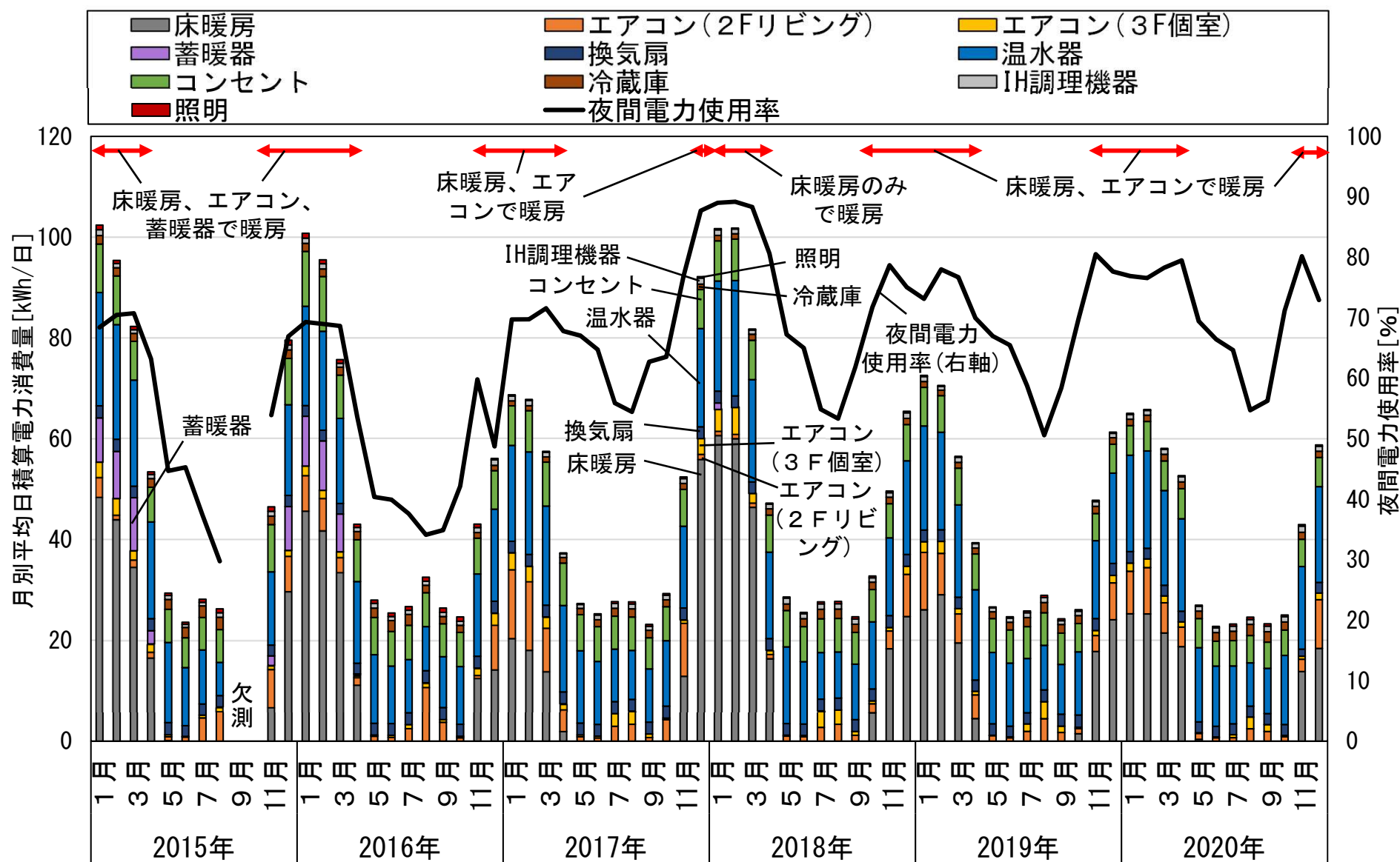
図4 用途ごとの月別平均日積算電力消費量
