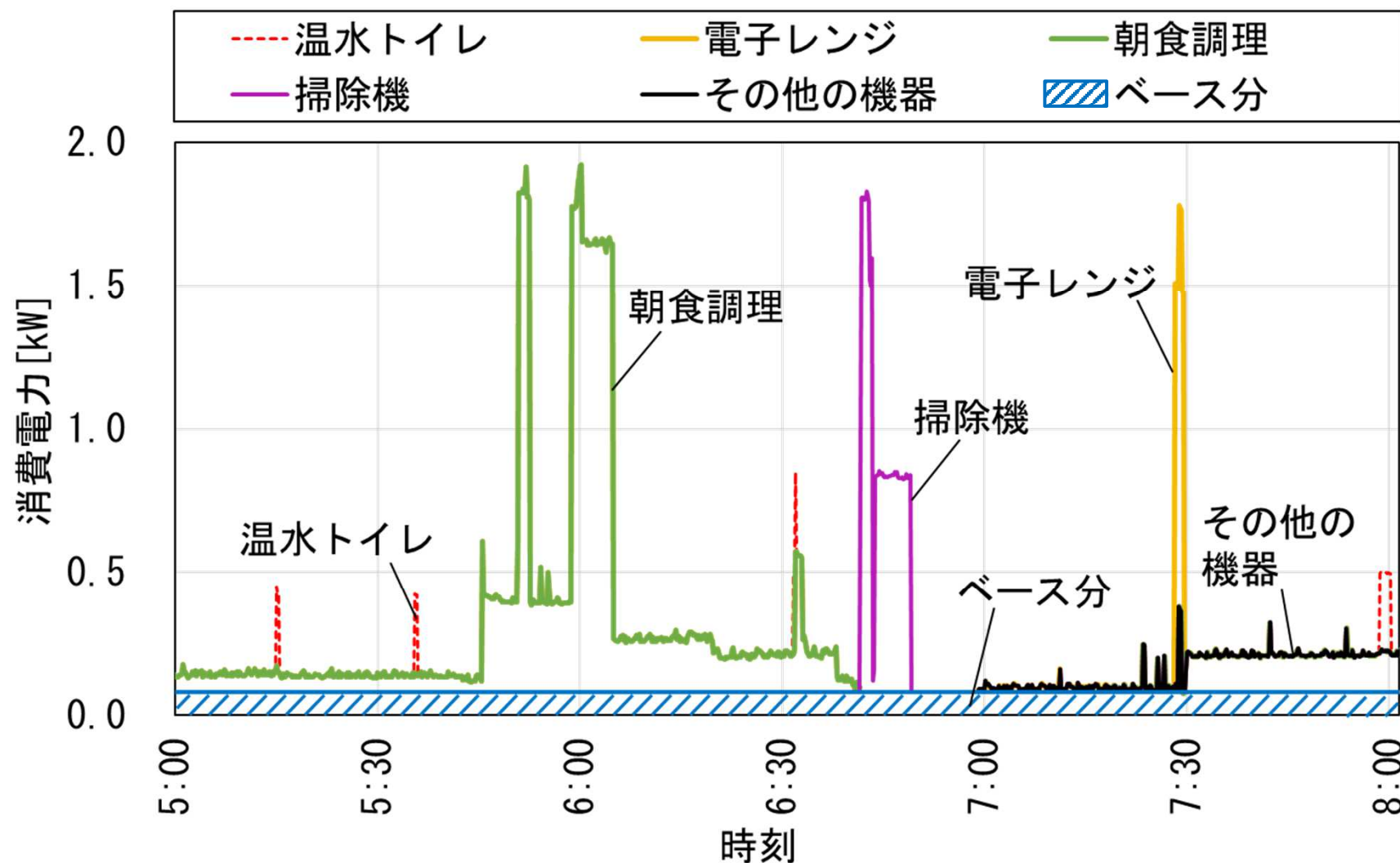
図3 コンセント系統の電力消費量 (2020年5月27日5:00~8:00)
