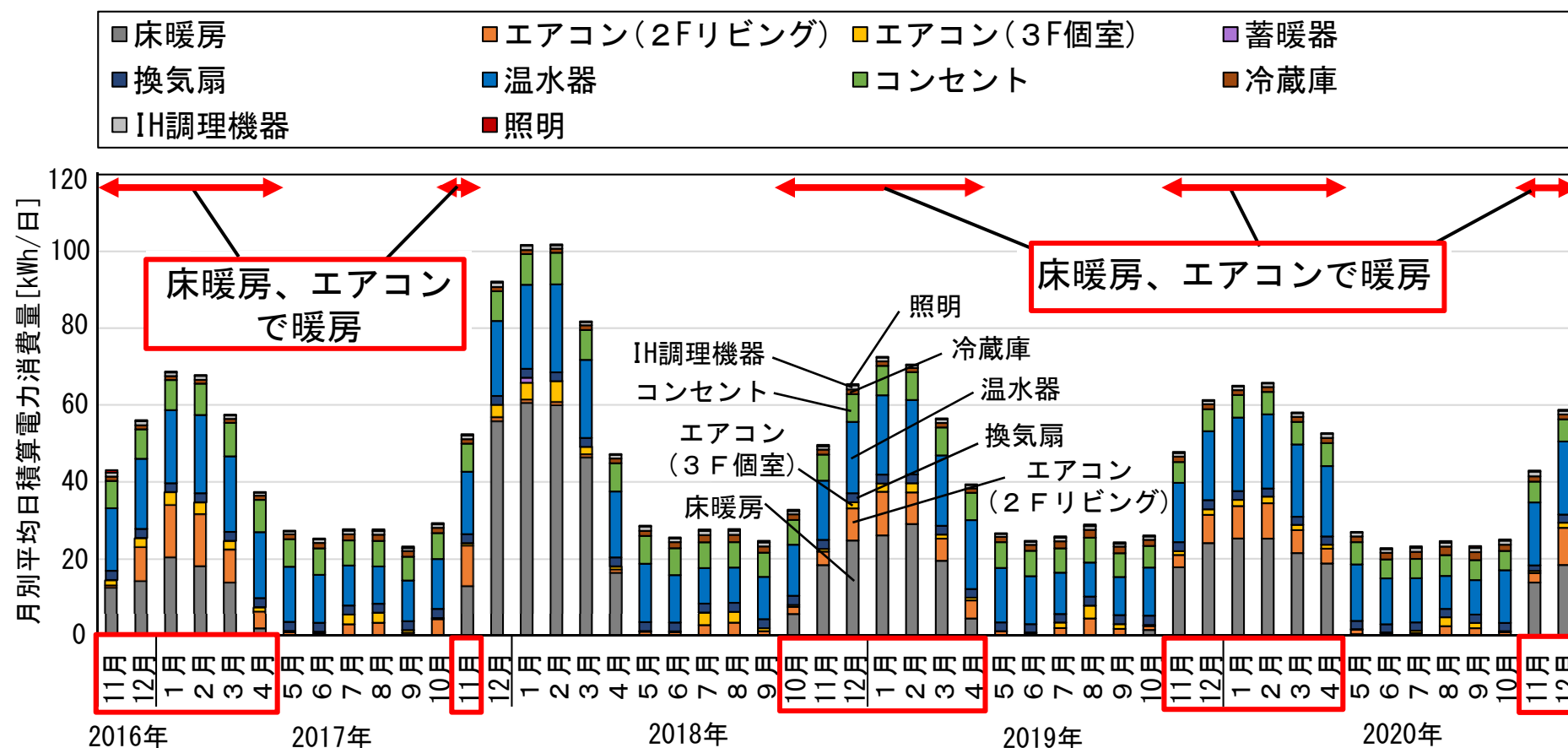
図 用途ごとの月別平均日積算電力消費量(2016年11月～2020年12月)
