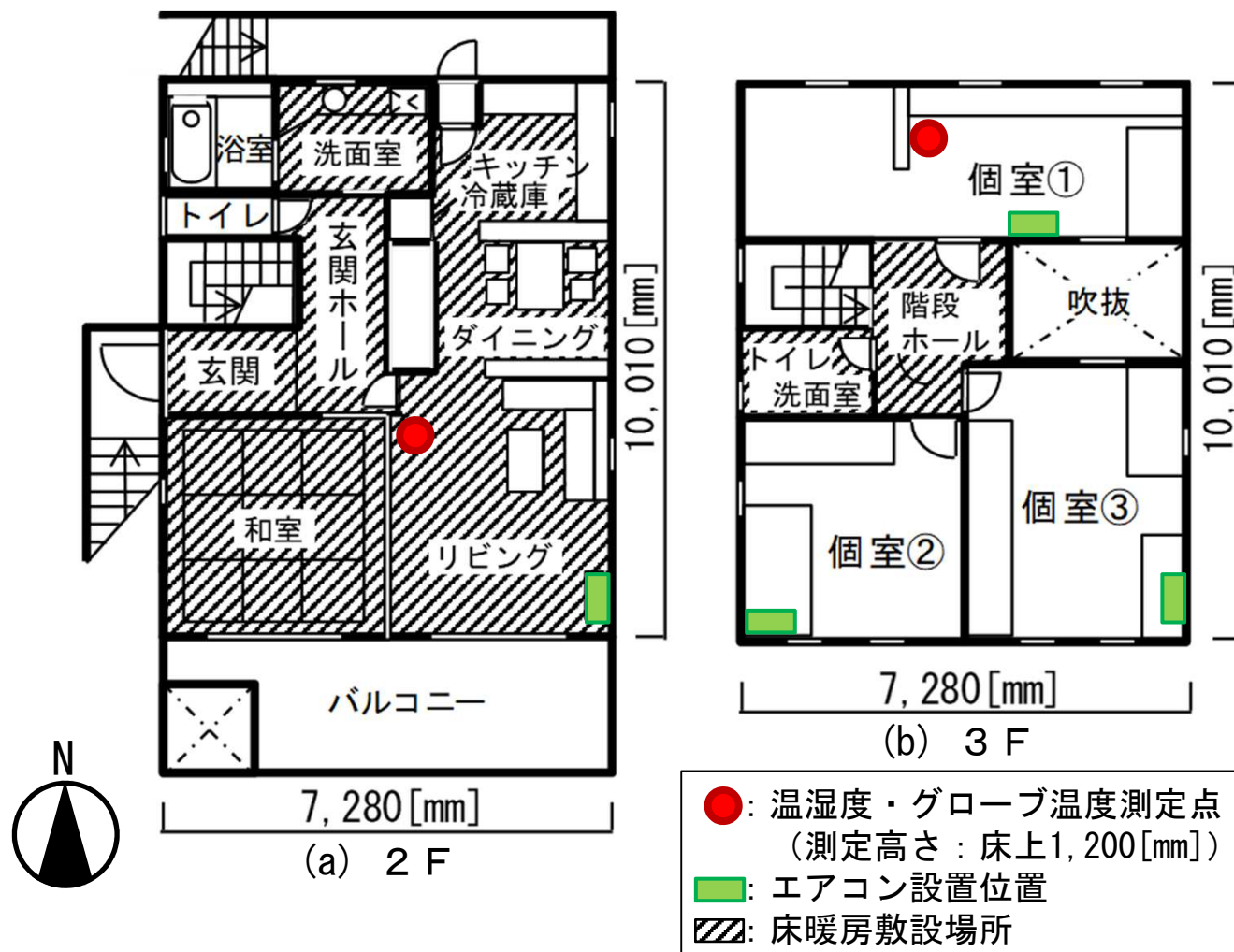
図1 対象住宅の平面※1
