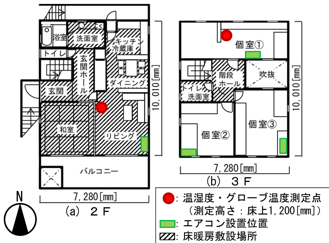
図1 対象住宅の平面※1
