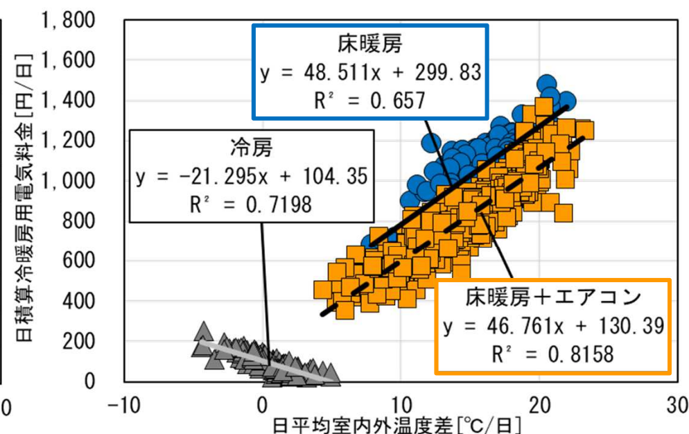
(b) 日積算冷暖房用電気料金と 日平均室内外温度差の関係
