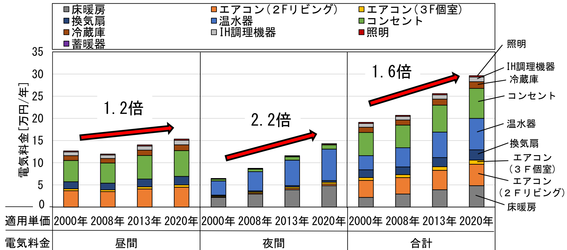
図 6 2019年度の電力消費量を基にした各年度の電気料金単価に対応した年積算電気料金
